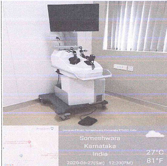
1.Laparoscope trainer
